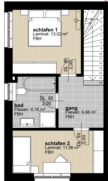
Wohnungsgrundriss Obergeschoss
