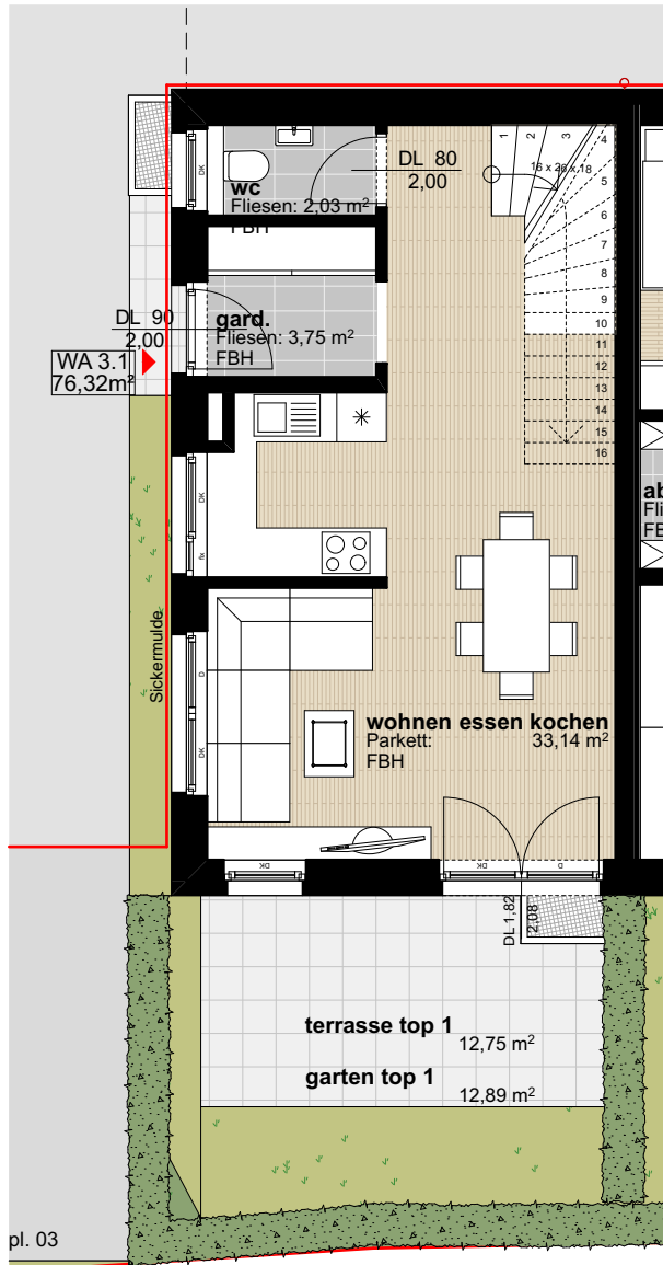
Wohnungsgrundriss Erdgeschoss
