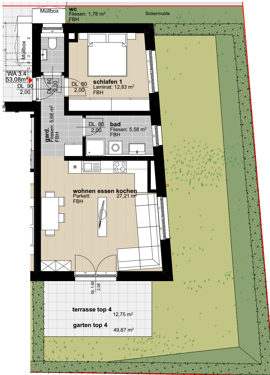
Wohnungsgrundriss
